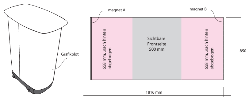
Grafikmasse für Expand PodiumCase als Theke
