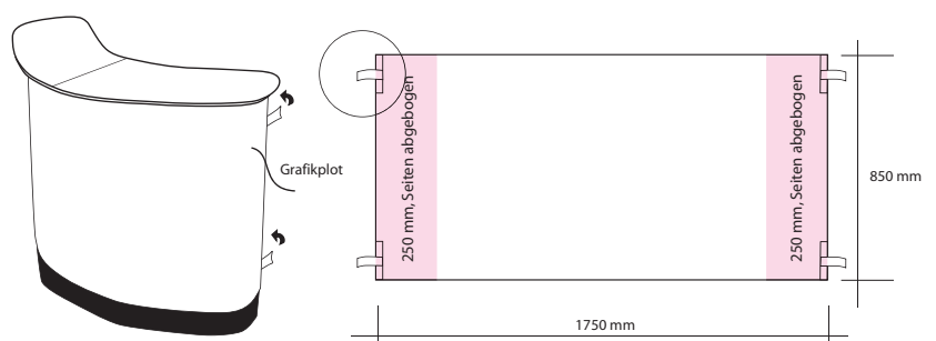
Grafikmasse für Expand PodiumCase als Theke
